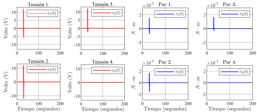
Figura 5.14: Caso 2: Tensión aplicada a las ruedas de reacción y par generado.
