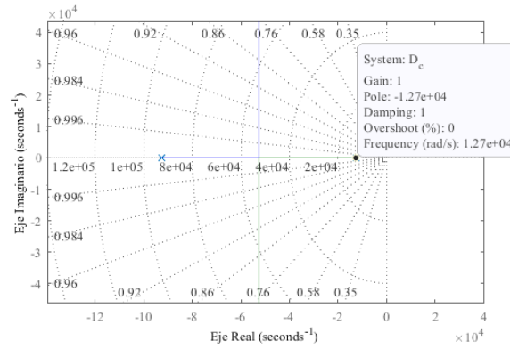
Figura 5.4: Lugar de las raíces de la función de transferencia D_c(s) si C_d(s) = 0.00001 .
