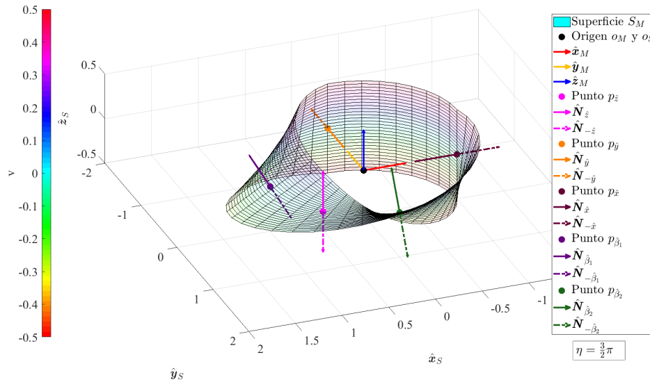
Figura 4.14: Banda de Möbius modificada con \eta = 3/2\pi .
